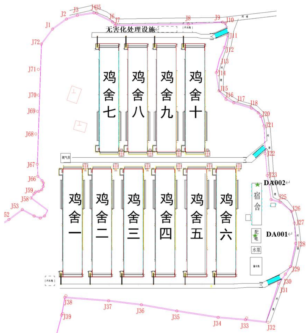
图 3.1-1：项目总平面布置图示意图
