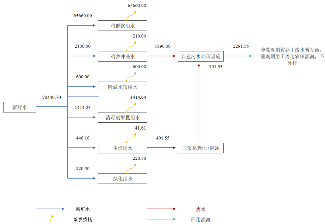
图 3.3-1：项目营运期水平衡图 (m³/a)
