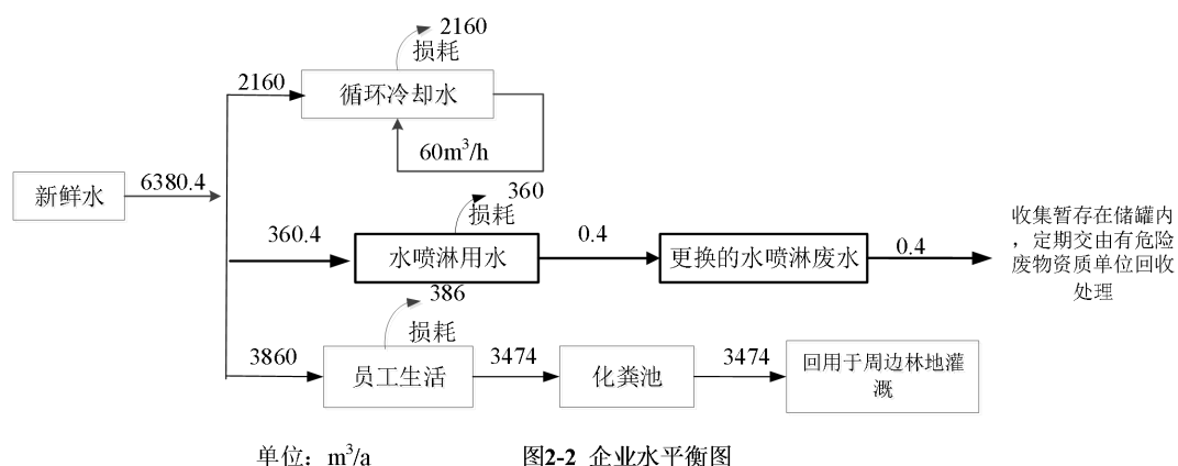
图2-2 企业水平衡图
