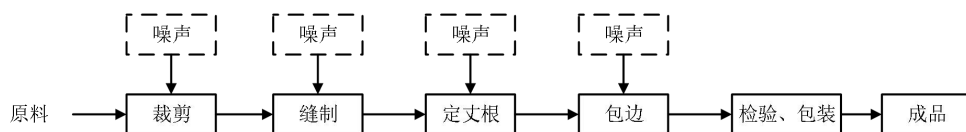
图2-6 项目营运期眼罩生产工艺流程及产污环节图
