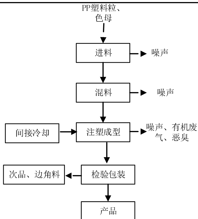
图2-4项目营运期一次性塑料杯生产工艺流程及产污环节图
