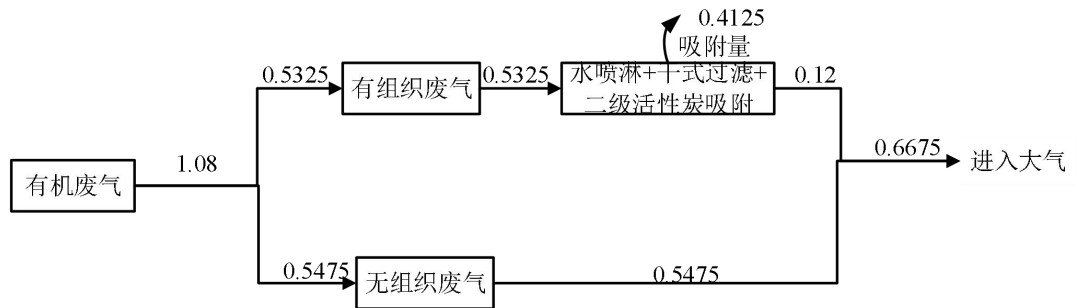
图2-1 注塑、热压、贴合工序的有机废气平衡图 单位t/a
